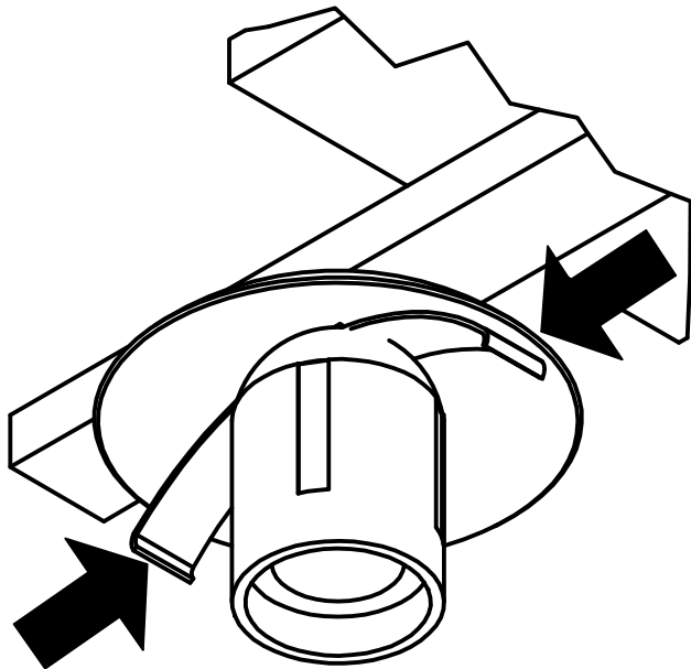
Detalhe "A"
